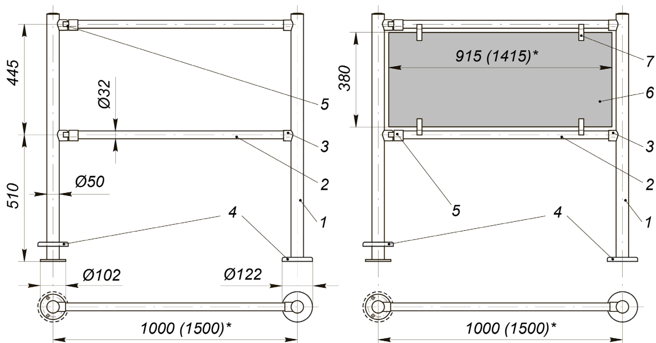
Рисунок 3. Секция ограждения без заполнения с поворотными патрубками 1 : 1 – стойка BH02 2-00(01,02,03); 2 – поручень BH02 1-00(01); 3 – патрубок BH02 0-10; 4 – декоративная крышка на фланец (в комплекте стоек ограждения); 5 – патрубок поворотный BH02 0-11, 6 – заполнение (тонир. стекло или полимерный материал); 7 – держатель BH02 0-02
