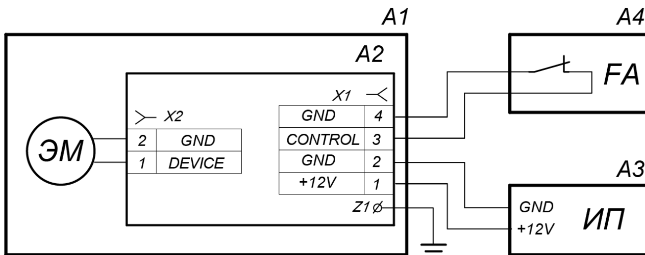
Рисунок 18. Схема электрических соединений при подключении стойки с электромагнитным УБ
